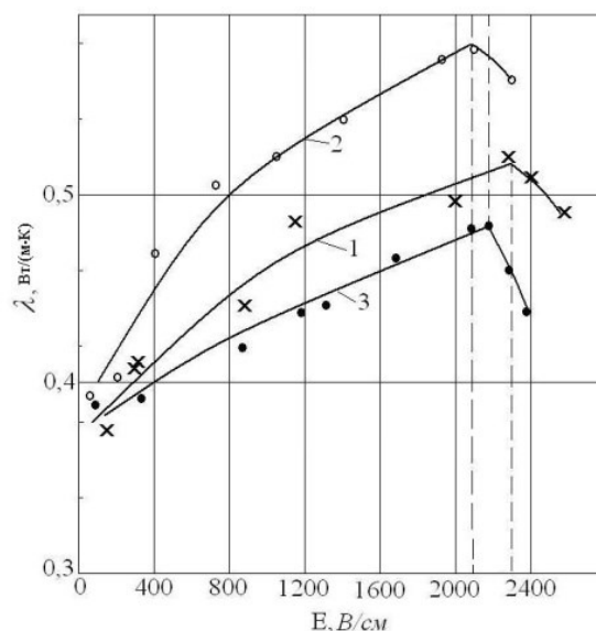
Рисунок 1 – Зависимость коэффициента теплопроводности электрообработанных полимерных прокладок с дисперсным наполнителем в виде алюминиевой пудры – 1, алюминиевой пудры, обработанной в растворителе – 2 и окисленного медного порошка – 3 от напряженности постоянного электрического поля.
