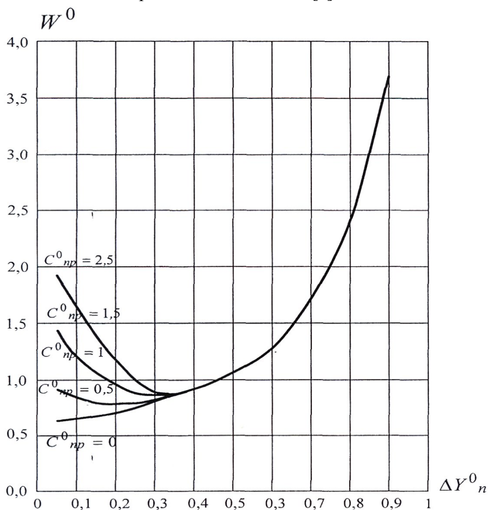
Рисунок 1 – Изменение издержек ремонтного обеспечения элемента W^0 в зависимости от величины упреждающего допуска \Delta Y_n^0 и потерь от простоя C_{np}^0
