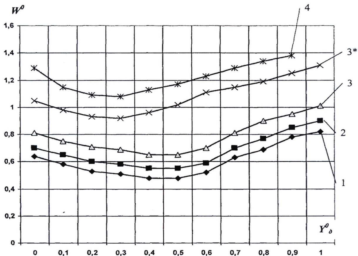
Рисунок 3 – Зависимость нормированных издержек ремонтного обеспечения элементов W^0 от допустимого отклонения параметра состояния Y^0 и варианта описания их непрерывной составляющей
