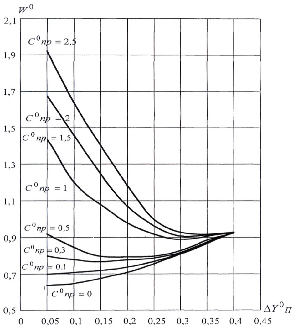
Рисунок 2 – Изменение издержек ремонтного обеспечения элемента в зависимости от величины упреждающего допуска \Delta Y_n^0 и потерь от простоя C_{np}^0
